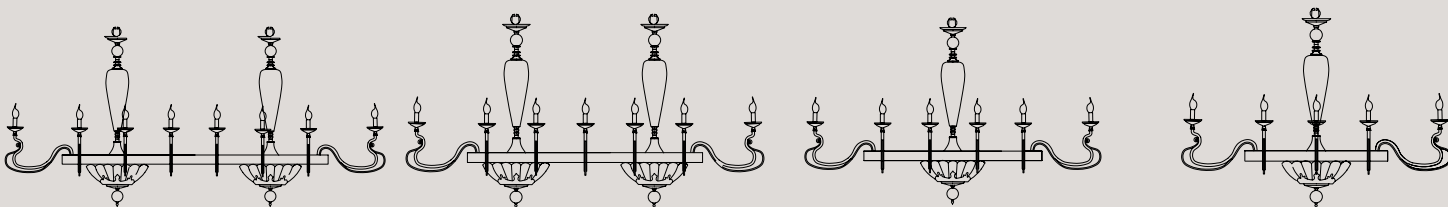
Barocco Axis 14 14 E14 x 40W 166x76 cm - H 90 cm
