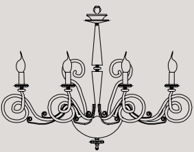
L6 6 E14 x 40W Ø 77 cm - H 85 cm
