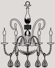
L5 5 E14 x 40W Ø 65 cm - H 80 cm
