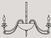
A2 2 E14 x 40W 40x26 cm - H 42 cm
