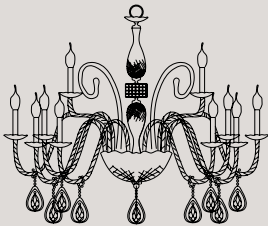
L12+6+6 24 E14 x 40W Ø 110 cm - H 80 cm
