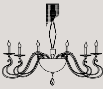
L8 8 E14 x 40W Ø 80 cm - H 70 cm
