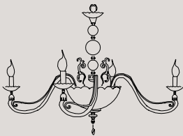
L5 5 E14 x 40W Ø 78 cm - H 80 cm
