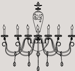
L8 8 E14 x 40W Ø 80 cm - H 70 cm
