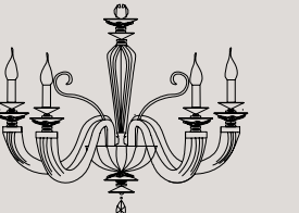
L6 6 E14 x 40W Ø 86 cm - H 73 cm
