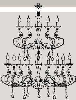
L12+6 LUX / 2 LEVELS 18 E14 x 40W Ø 80 cm - H 120 cm
